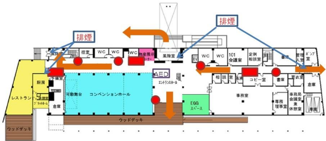
1階 避難経路
